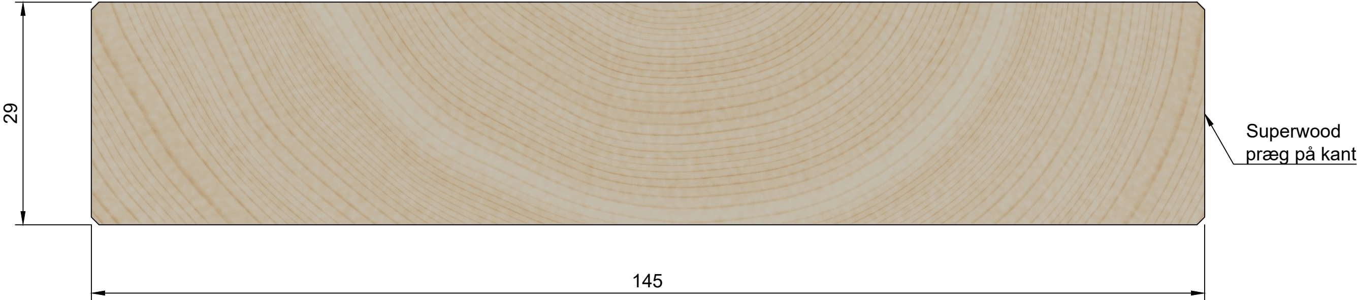
Ruhøvles 4 sider
